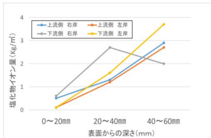
簡易測定法による塩化物イオン量の分布
