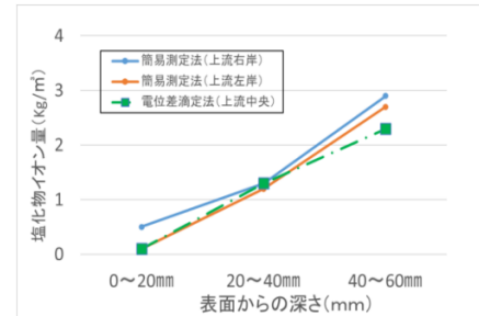
簡易測定法と電位差滴定法との比較
